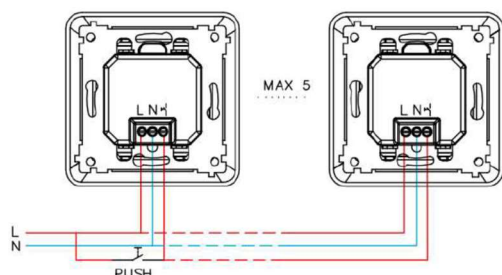
Yhden ovikellon yhden painikkeen (tai enintään viiden) kytkentäkaavio
