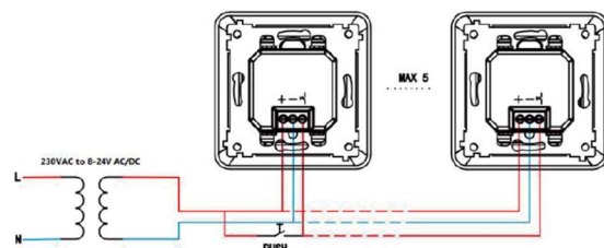
Enintään viiden ovikellon yhteisen painikkeen kytkentäkaavio
