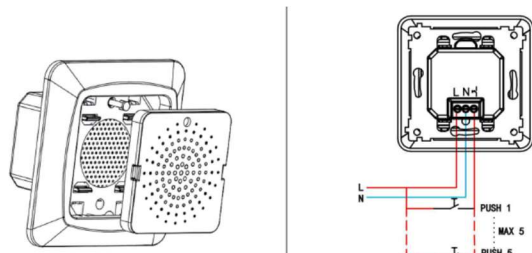
Yhden ovikellon yhden painikkeen (tai enintään viiden) kytkentäkaavio
